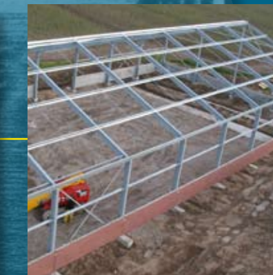
Stalen gordingen
